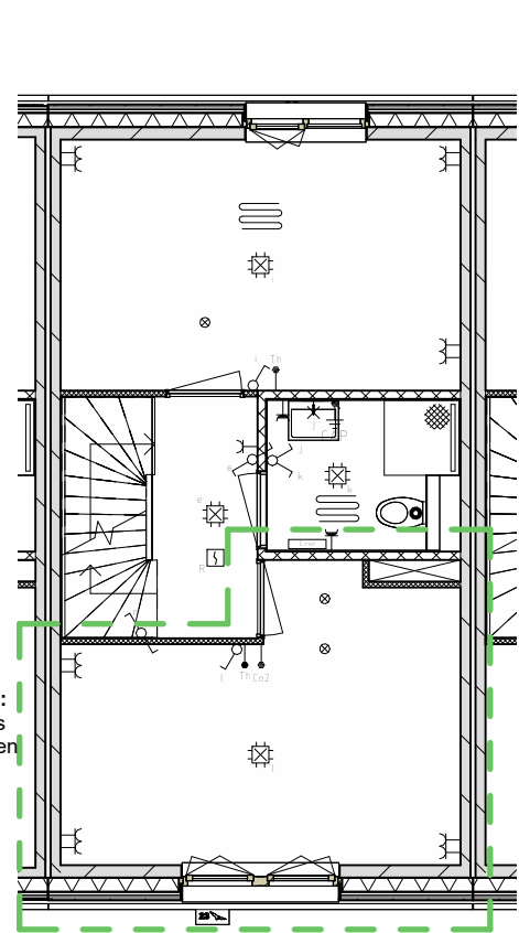
eerste verdieping
