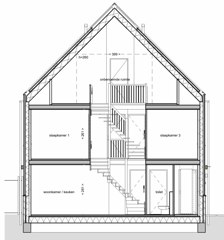
doorsnede
