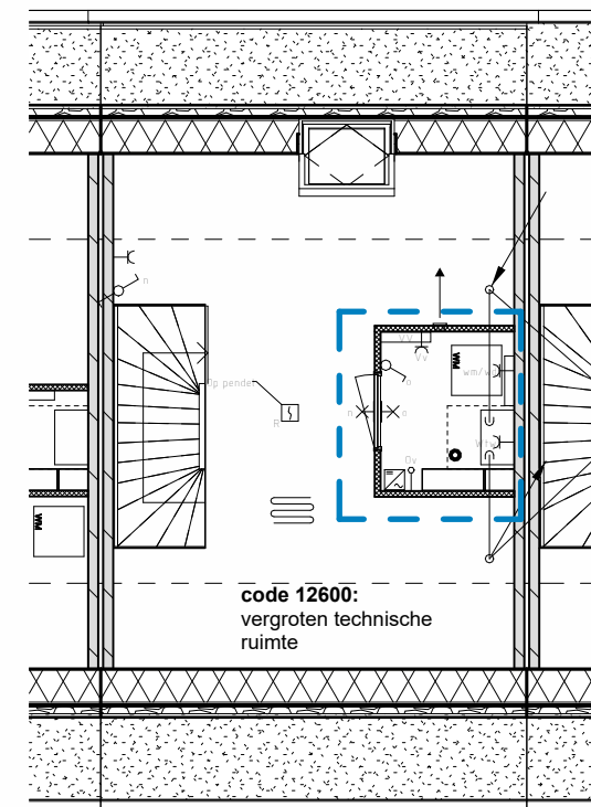
tweede verdieping
